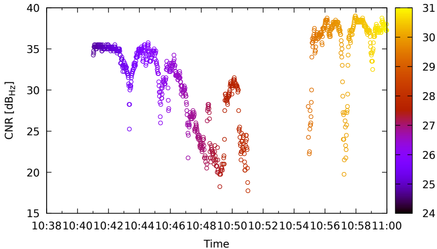
Timeline for E15 (E1) on XiaomiMi8 - DOY 262
