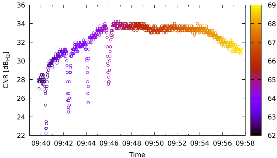
Timeline for E10 (E5a) on SamsungS20 - DOY 263
