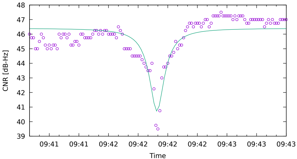
CNR fit for E10 on SamsungS20 - drive 2 (DOY263)
