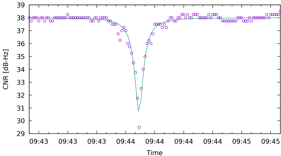
CNR fit for E10 on XiaomiMi8 - drive 3 (DOY263)
