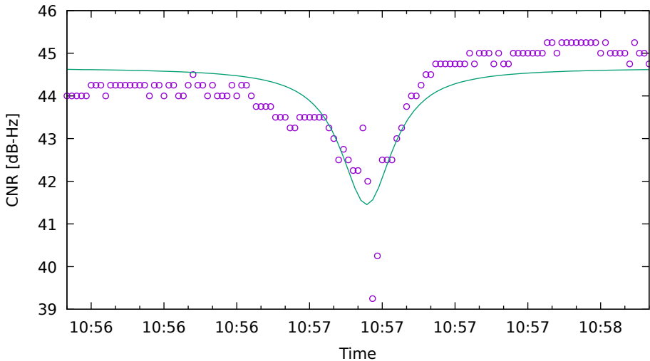
CNR fit for E10 on SamsungS20 - drive 10 (DOY263)
