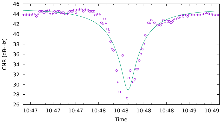
CNR fit for E10 on SamsungS20 - drive 5 (DOY263)
