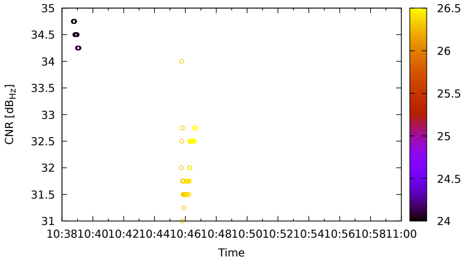
Timeline for E15 (E1) on Xiaomi11T - DOY 262
