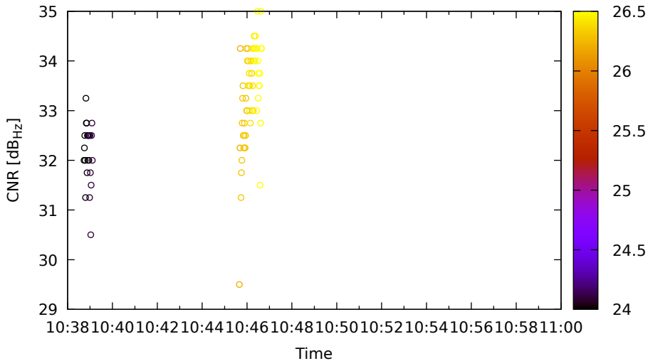
Timeline for E15 (E5a) on Xiaomi11T - DOY 262
