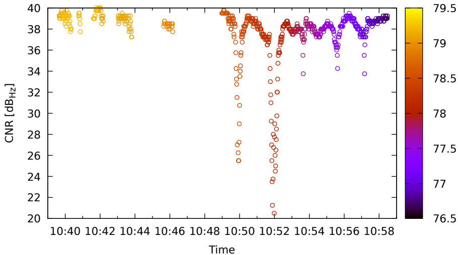
Timeline for E10 (E1) on Xiaomi11T - DOY 263
