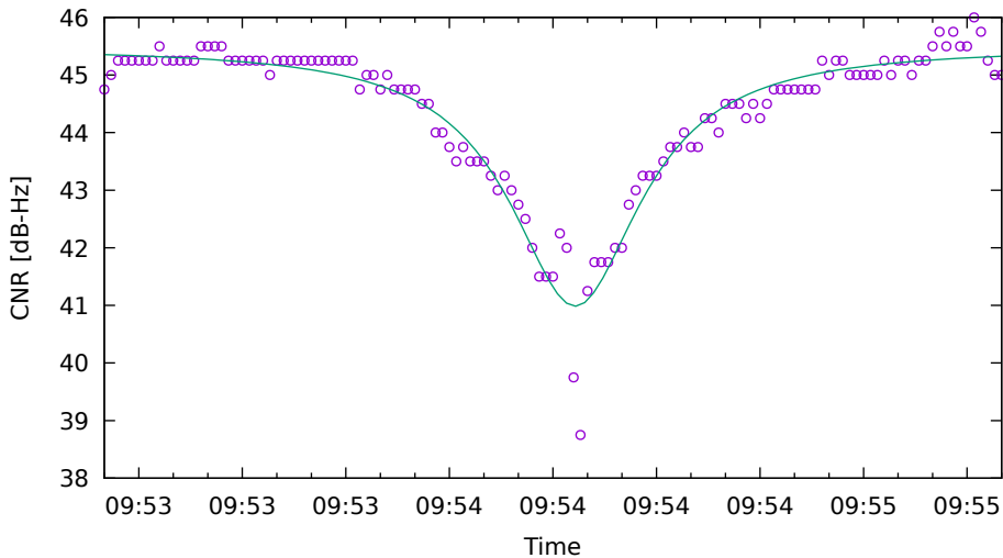
CNR fit for E10 on SamsungS20 - drive 9 (DOY263)
