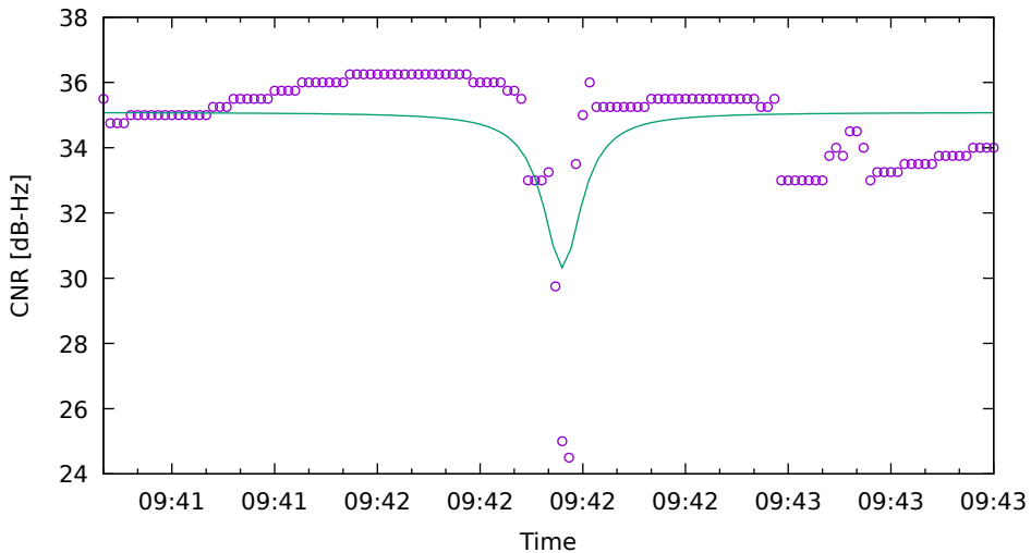
CNR fit for E10 on Xiaomi11T - drive 2 (DOY263)
