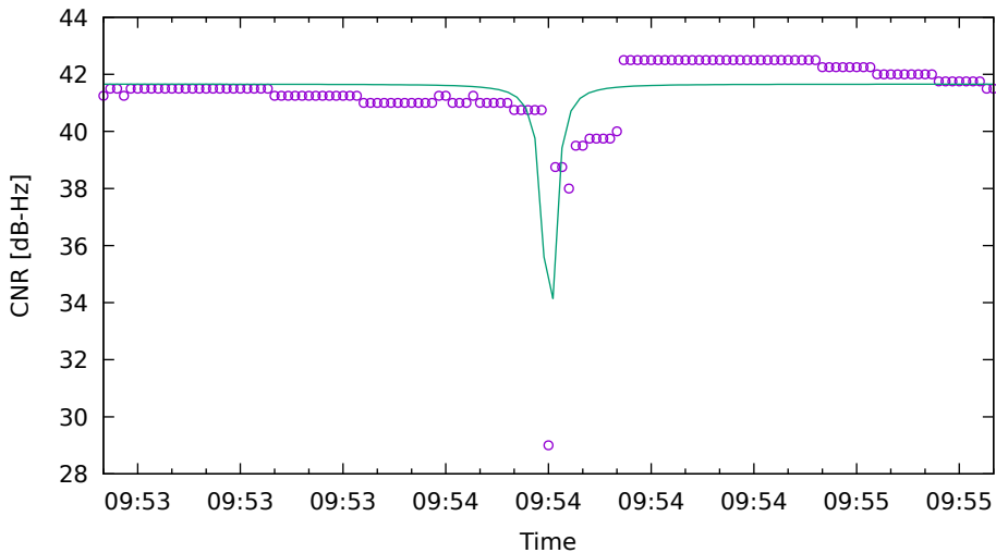
CNR fit for E10 on Xiaomi11T - drive 9 (DOY263)
