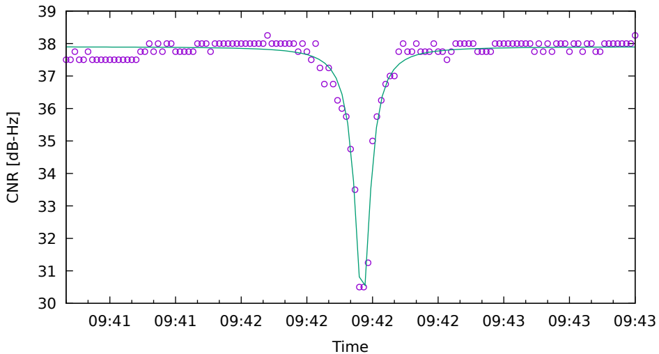
CNR fit for E10 on XiaomiMi8 - drive 2 (DOY263)
