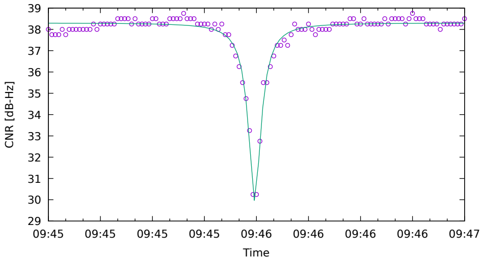
CNR fit for E10 on XiaomiMi8 - drive 4 (DOY263)
