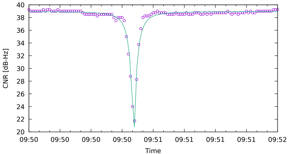
CNR fit for E10 on XiaomiMi8 - drive 7 (DOY263)
