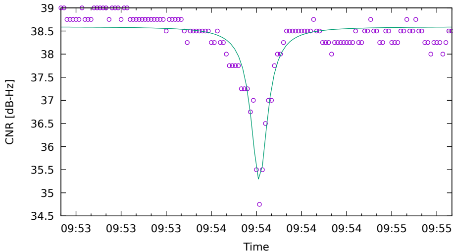
CNR fit for E10 on XiaomiMi8 - drive 9 (DOY263)
