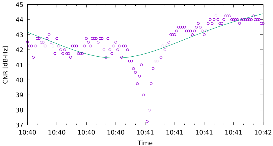
CNR fit for E10 on SamsungS20 - drive 1 (DOY263)
