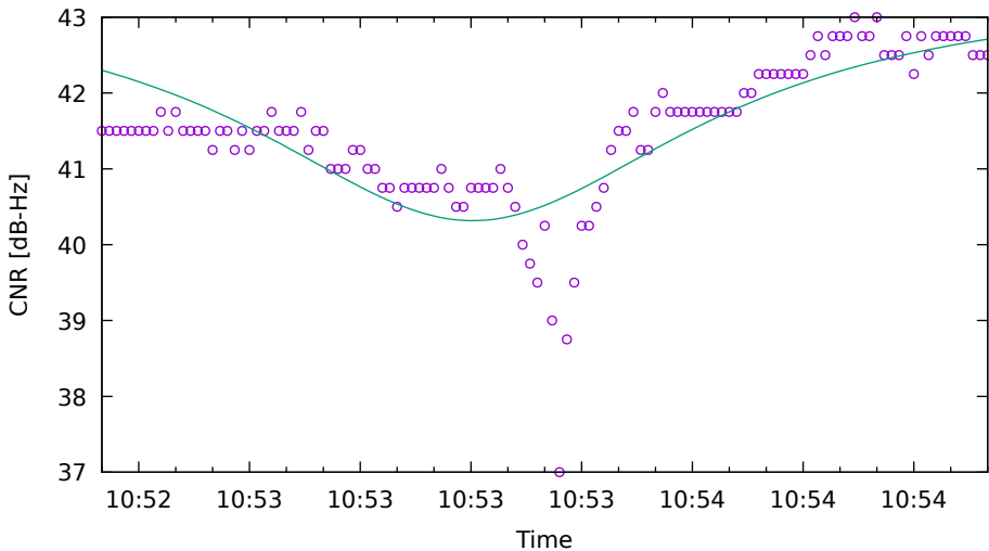
CNR fit for E10 on SamsungS20 - drive 8 (DOY263)
